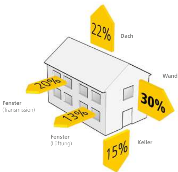
Durchschnittliche Wärmeverluste eines Mehrfamilienhauses
